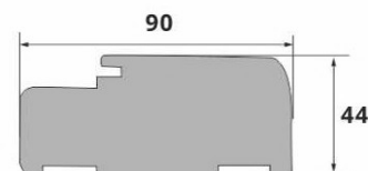
przekrój ościeżnicy stałej
